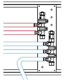
Udsnit A - Fordeletrør (3K/2V) Mål: 1 : 10
